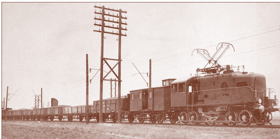
Az első fázisváltós próbamozdony egyik útján, Dunakeszi-Alag és Rákosrendező között. Fojtán István gyűjteményéből
